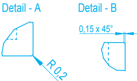
Sichtkanten - Profil
