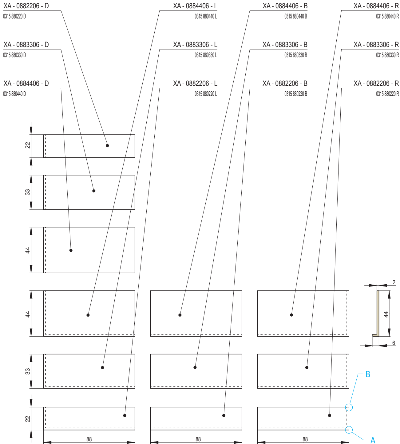
Sichtkanten - Profil
