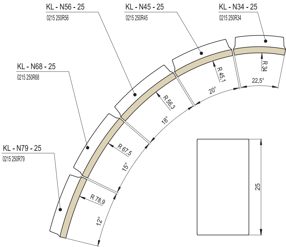
Höhe 25 cm
