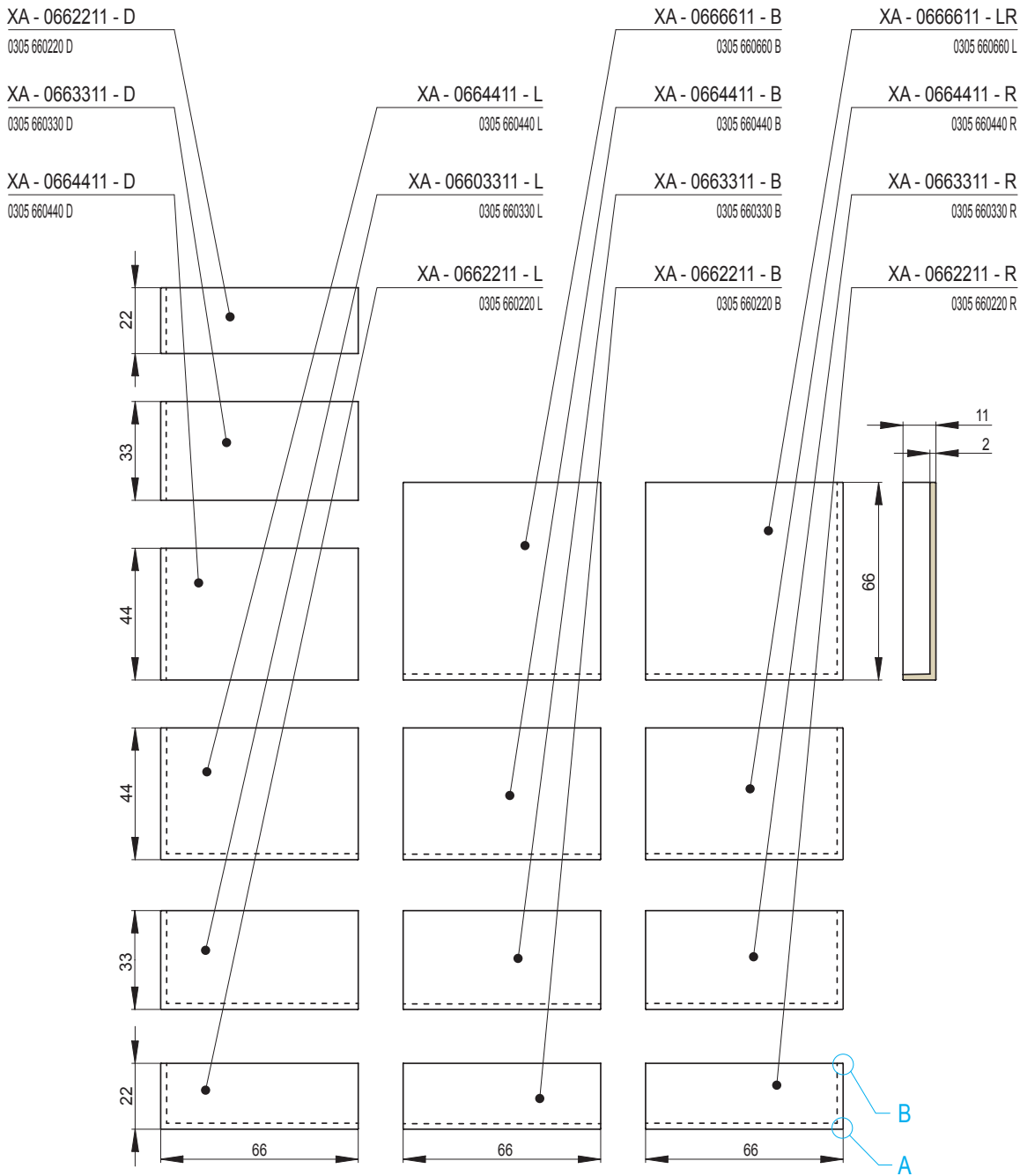
Sichtkanten - Profil
