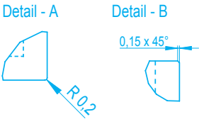
Sichtkanten - Profil
