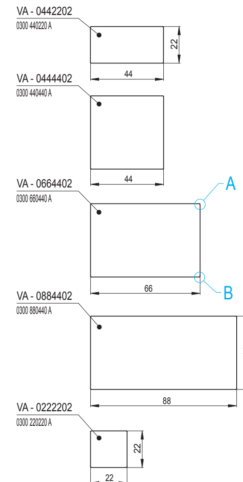
Sichtkanten - Profil
