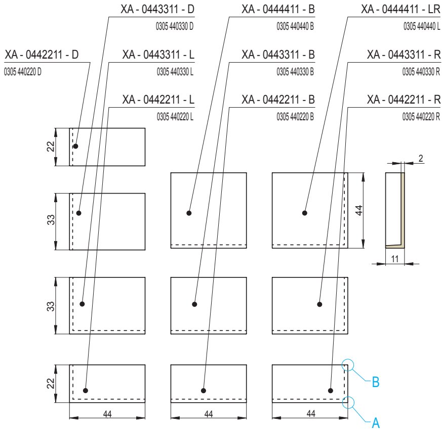
Sichtkanten - Profil
