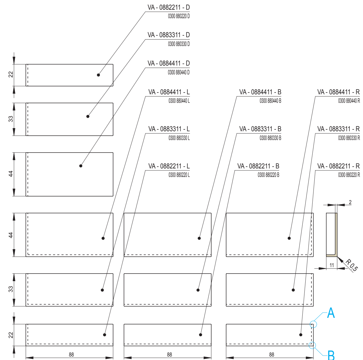
Sichtkanten - Profil
