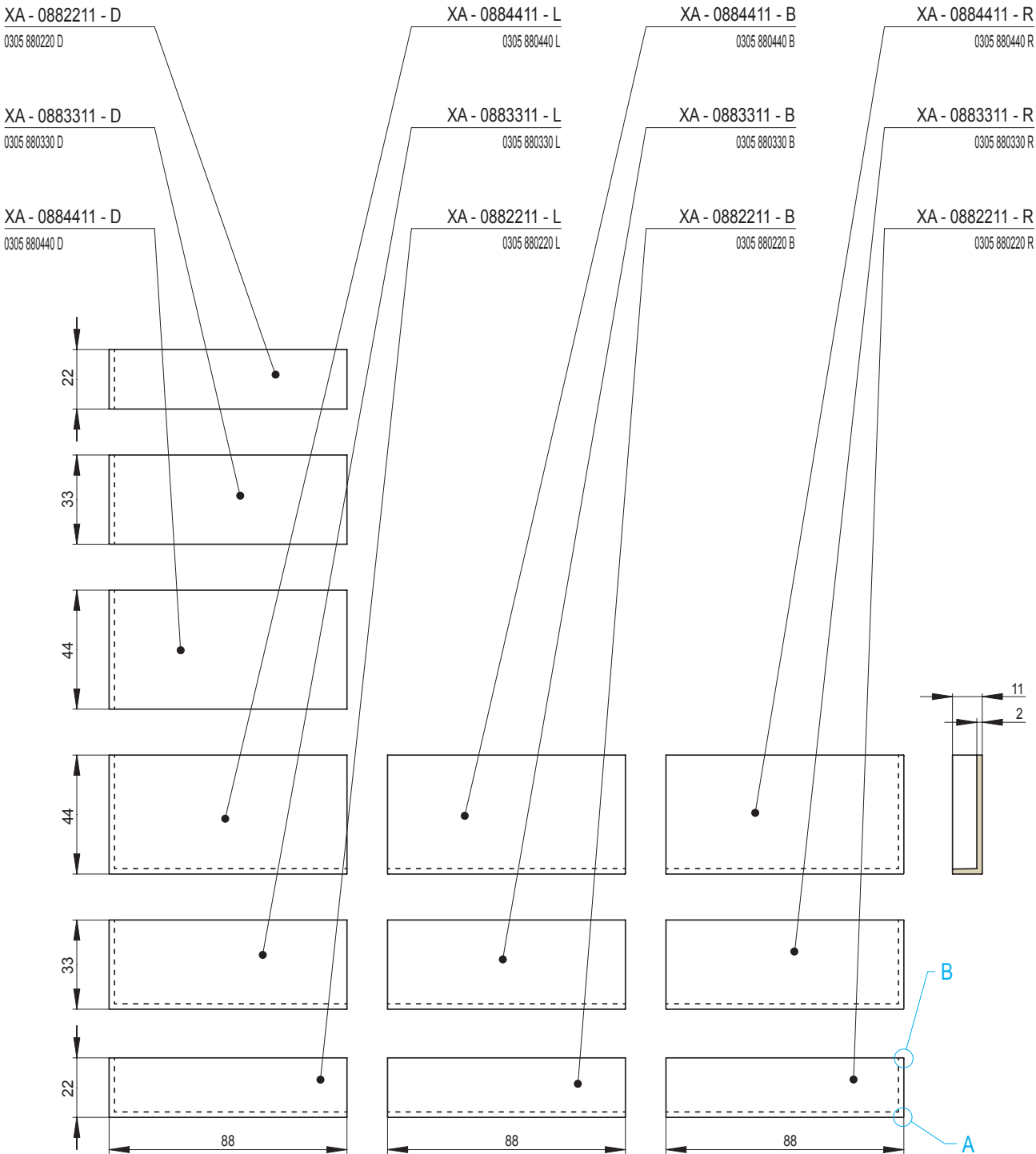
Sichtkanten - Profil
