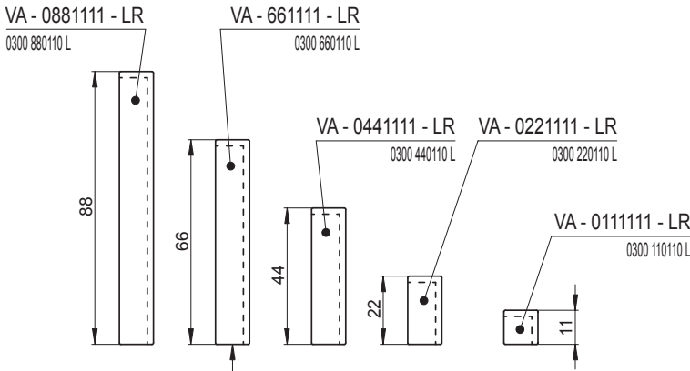
Seitenansicht
