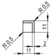
Seitenansicht
