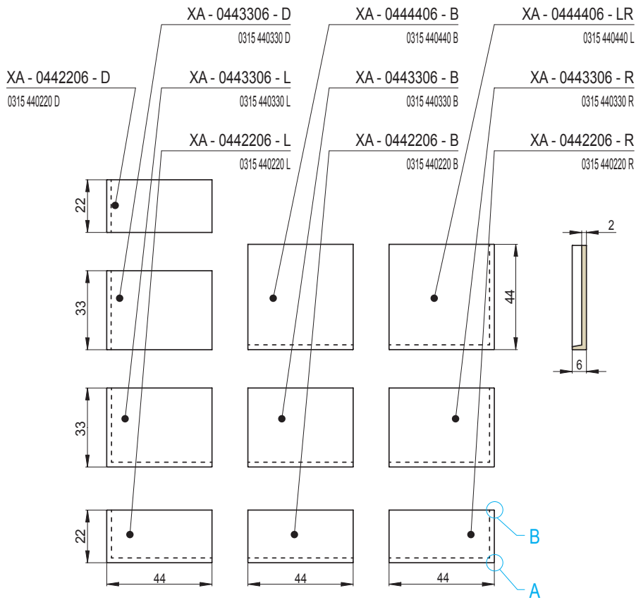
Sichtkanten - Profil
