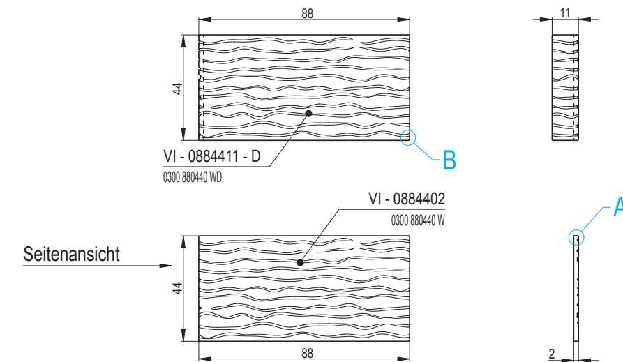
Sichtkanten - Profil
