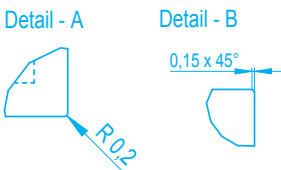
Sichtkanten - Profil
