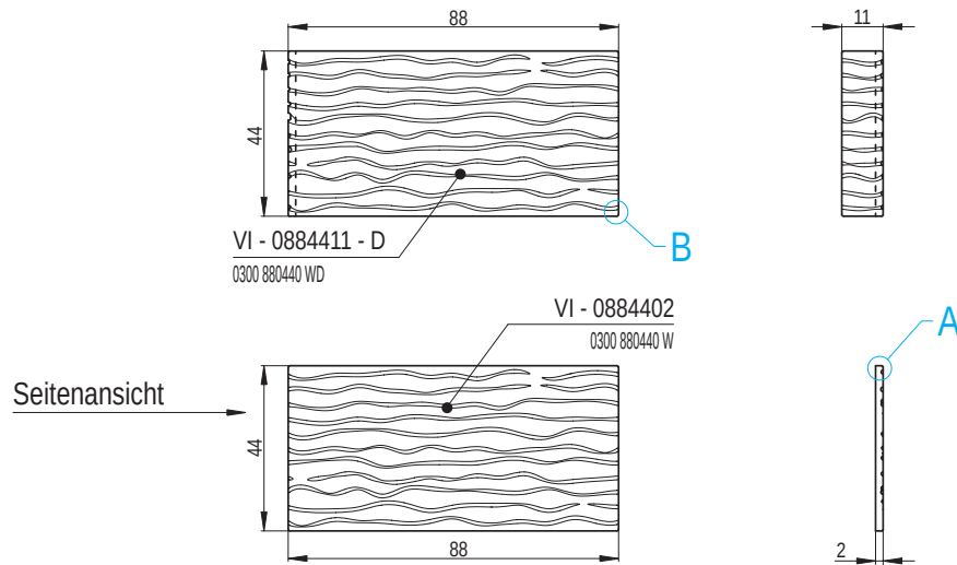
Sichtkanten - Profil
